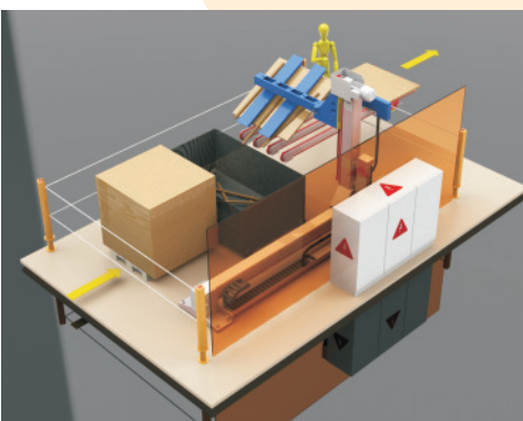
Lagenweise Beschickung mit Zwischenleistenabwurf
